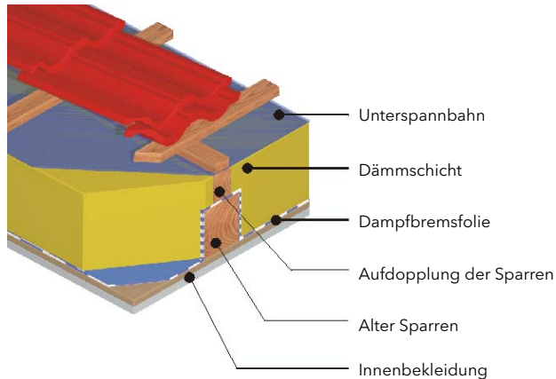
Schnitt durch ein Dach mit einer Dampfbremsefolie, die von außen um die Sparren herum geführt wurde
