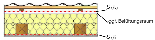
Dampfbremsewerte außen und innen
