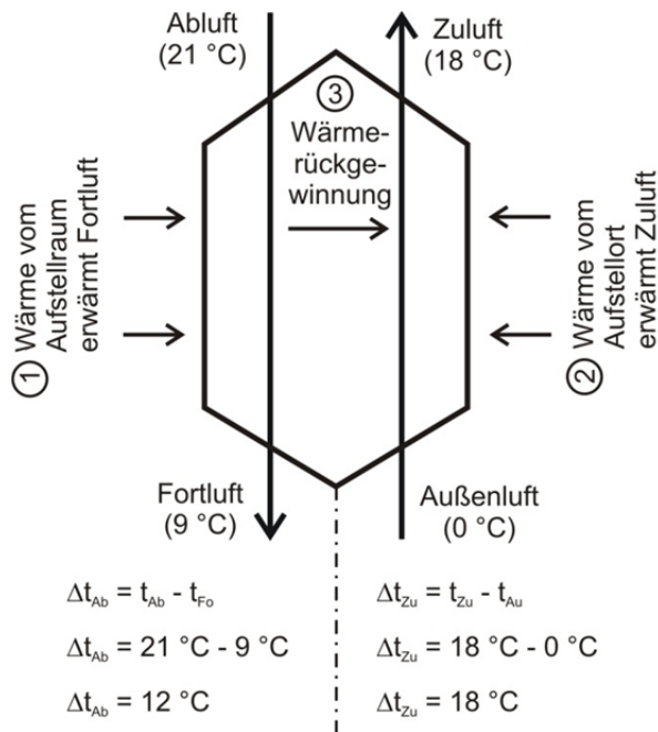
Bild 1: Einflussfaktoren auf die Lufterwärmung im WRG-Gerät
