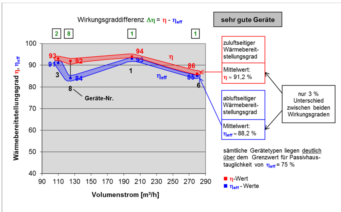
Bild 3: Bei guten Wärmerückgewinnungsgeräten gemessene Wärmebereitstellungsgrade ( \eta , \eta_{eff} ) mit nur geringfügigen Unterschieden
