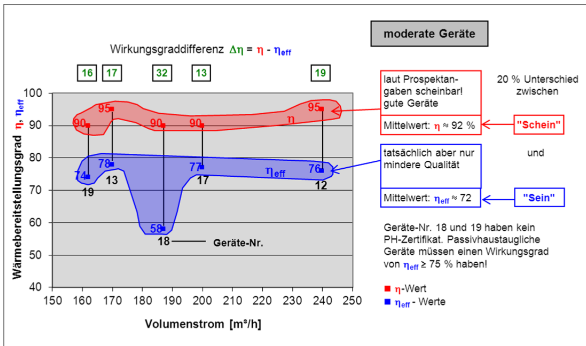
Bild 2: Bei weniger guten Wärmerückgewinnungsgeräten gemessene unterschiedliche Wärmebereitstellungsgrade:
