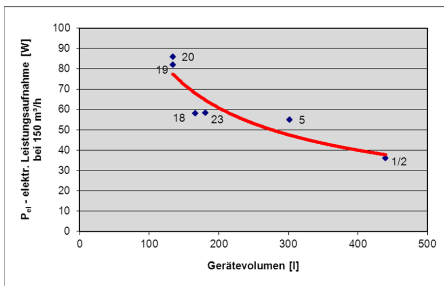
Bild 7: Abhängigkeit der Leistungsaufnahme vom Gerätevolumen
