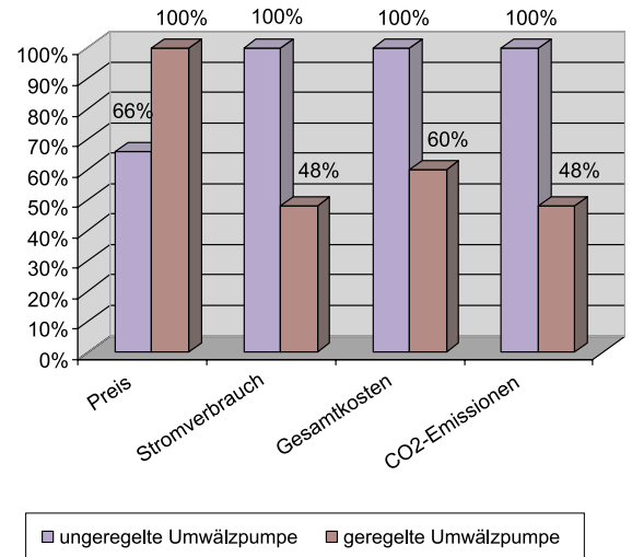
Abb. 19: Einsparmöglichkeit durch den Einsatz elektronisch geregelter Umwälzpumpen; Quelle: Grundfos GmbH, Wahlstedt
