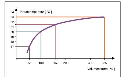
Abb. 17: Auswirkung des Volumenstroms auf die Raumtemperatur bei konstanter Heizfläche
